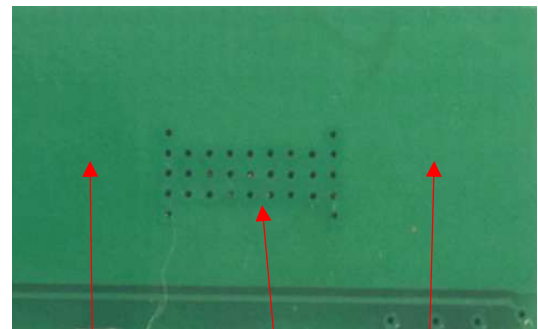
Large Cu area Thermal vias Large Cu area
