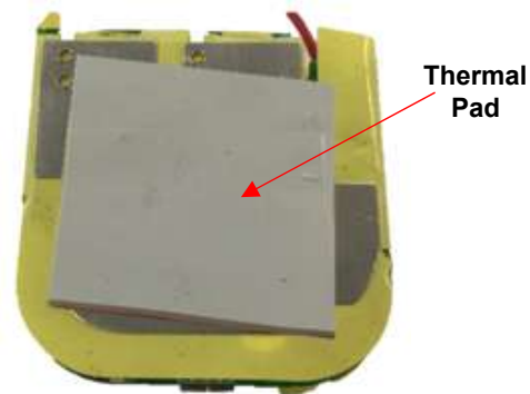
(d) Place thermal pad over aluminum sheet
