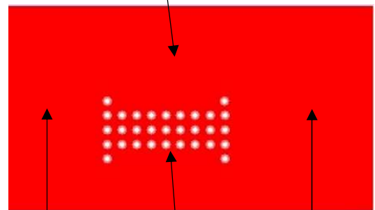
Large Cu area Thermal vias Large Cu area
